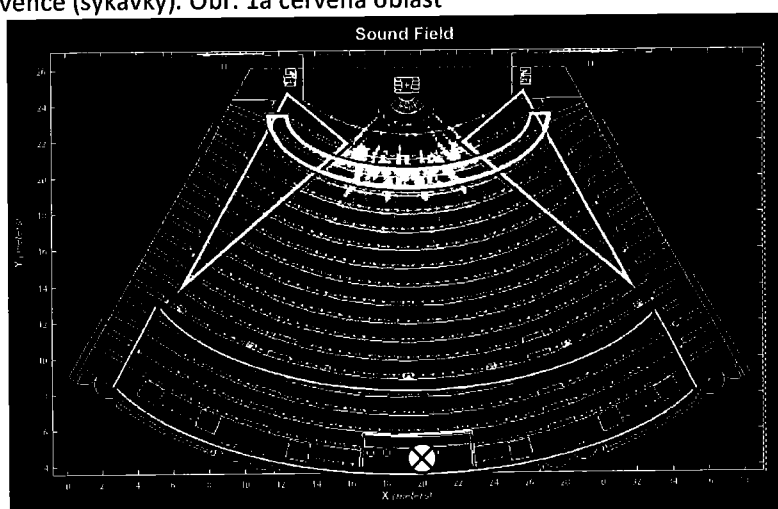
Obr. 1a VOCAL – současný stav. Center cluster JM-1P. „Hluchá“ místa jsou na obrázku tmavá, vyznačeny jsou zóny bez vysokých frekvencí – chybí prezence. Záznam zastavení znázorňuje pozici FOH zvukaře – live post. Zobrazená frekvence 8kHz. 3dB / colour
