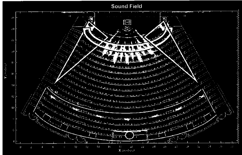
Obr. 2 VOCAL – výsledný stav, horizontální rovina . Central cluster JM-1P spolu s Filly vykryvá celé auditorium +/- 3dB. Smajlík označuje pozici FOH zvukaře. Zobrazená frekvence 8kHz. 3dB / colour.
