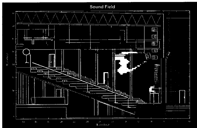
Obr.3 VOCAL – výsledný stav, vertikální rovina . Central cluster JM-1P spolu s Filly vykryvá celé auditorium +/- 3dB. Zelená čára označuje výšku uší posluchačů (minimum variance line), smajlík označuje pozici FOH zvukaře. Zobrazená frekvence 8kHz. 3dB / colour.
