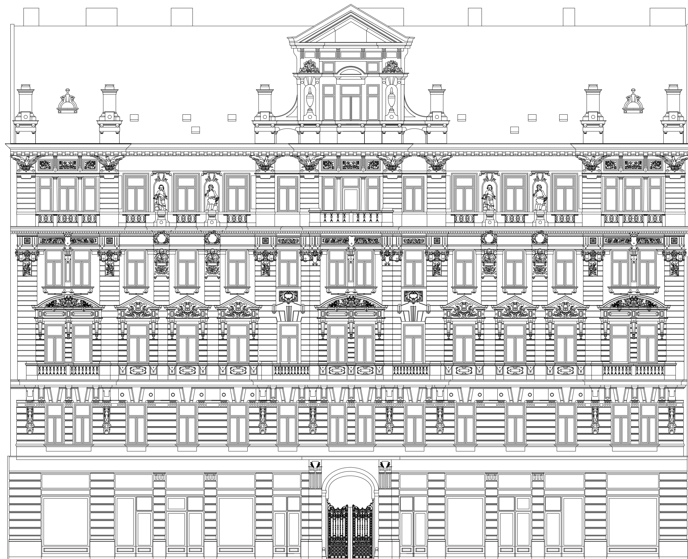
HISTORICKÝ STAV – POHLED NA "A" (ULICE) 1:125
